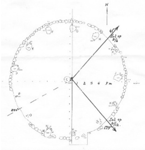
2. Stenkreds ved Andehøj. Tegningen i Havn Herold. (Opmålt og tegnet af H. Holten Andersen).
